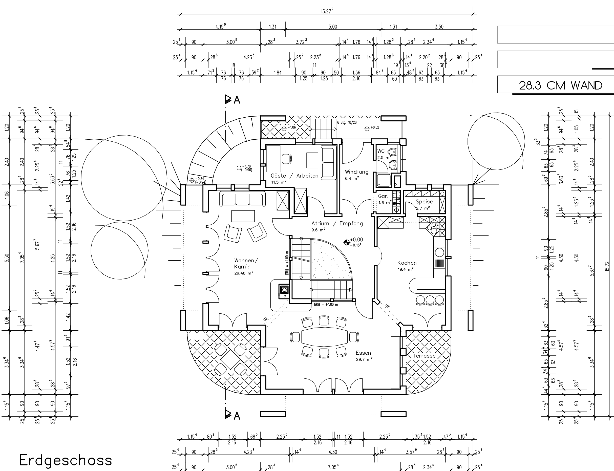
Erdgeschoss
